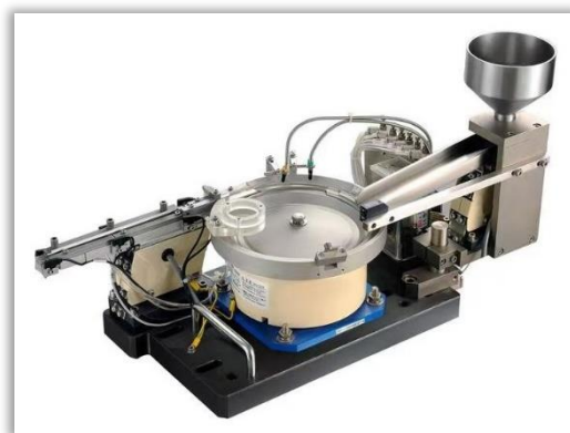
06 镍片振动盘
