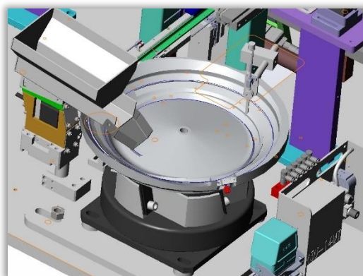
05 振动盘3D设计
