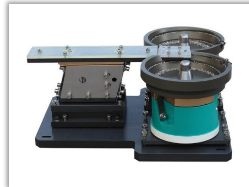
03 销钉振动盘
